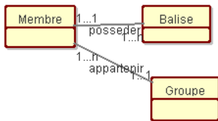
Fig. 2 : Métamodèle PIM
