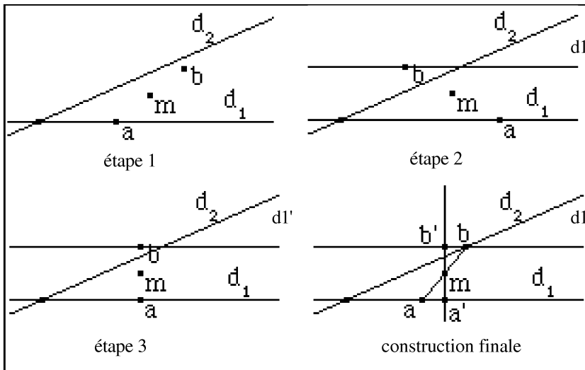
Figure 1 dessin d'un segment s'appuyant sur deux droites
