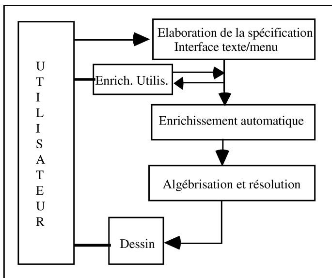
Figure 4 architecture de GéoSpécif et construction automatique
