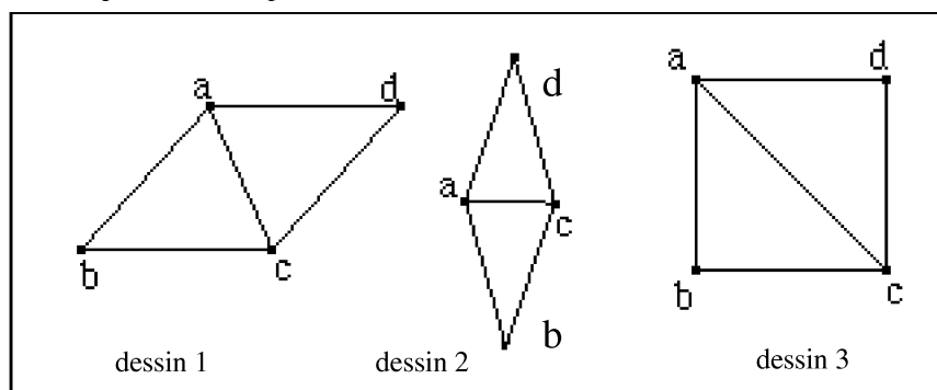
Figure 2 trois losanges obtenus à partir de triangles isocèles
