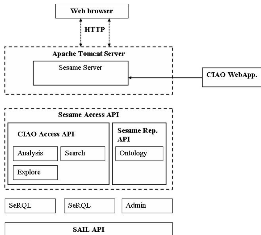
Figure 5.16 Architecture interne du système CIAO
