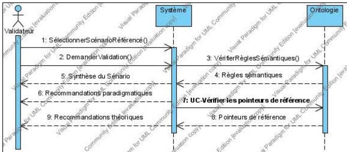
Figure 5.15 Diagramme de séquence lié au cas CU-3.2
