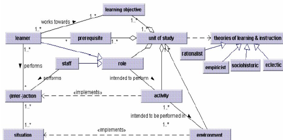
Figure 2.2 Le méta-modèle d'EML détaillé (en format UML)
