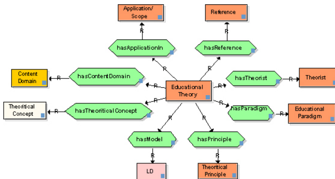
Figure 4.18 Modèle de propriétés du concept “Educational Theory” dans la sous-ontologie des TPAED
