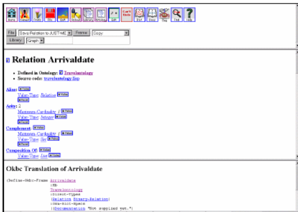
Figure 4.26 Interface principale d'Ontolingua
