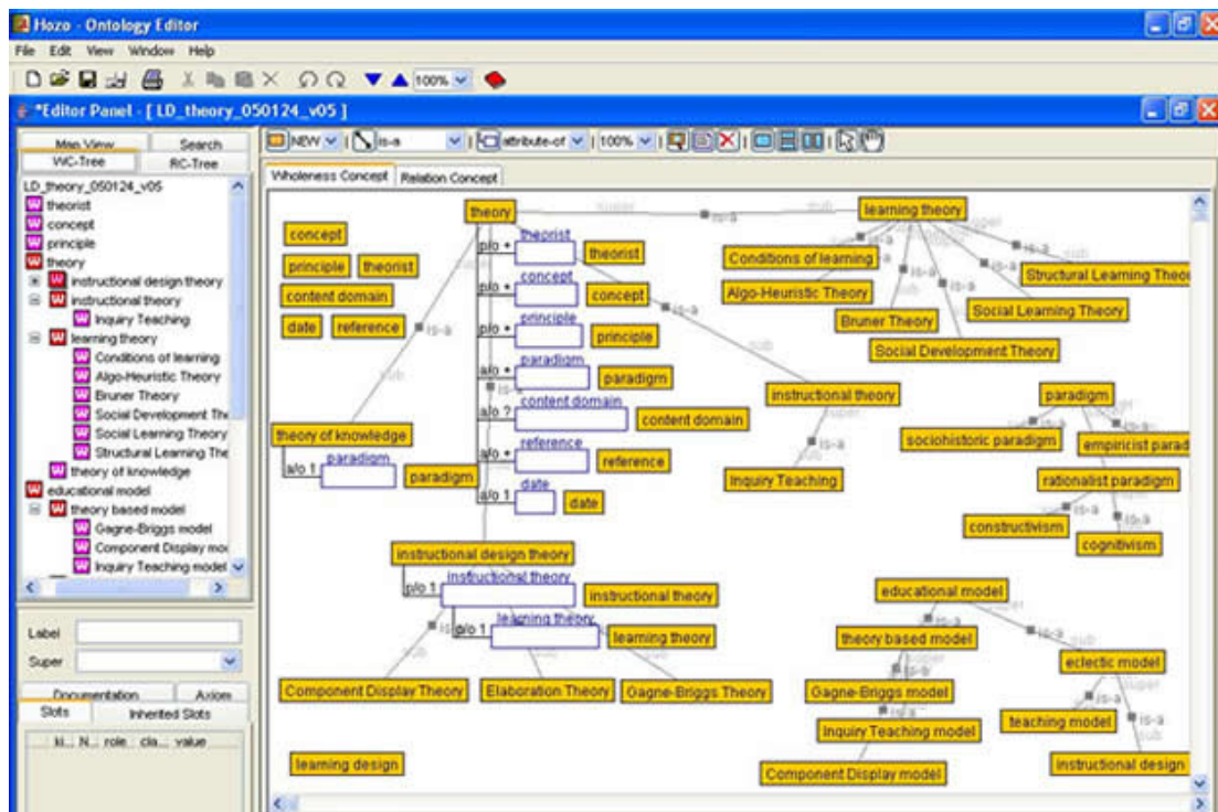
Figure 4.8 L'OTPAED intégrant EML et IMS-LD (dans Hoza)
