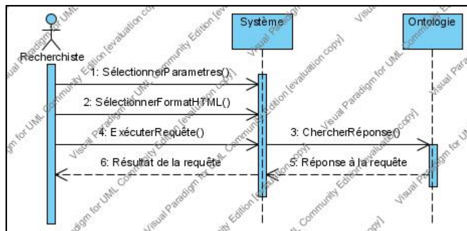
Figure 5.12 Diagramme de séquence lié au cas CU-2.2
