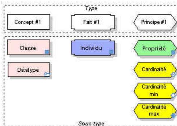
Figure G.9 Sous type d'élément OWL
