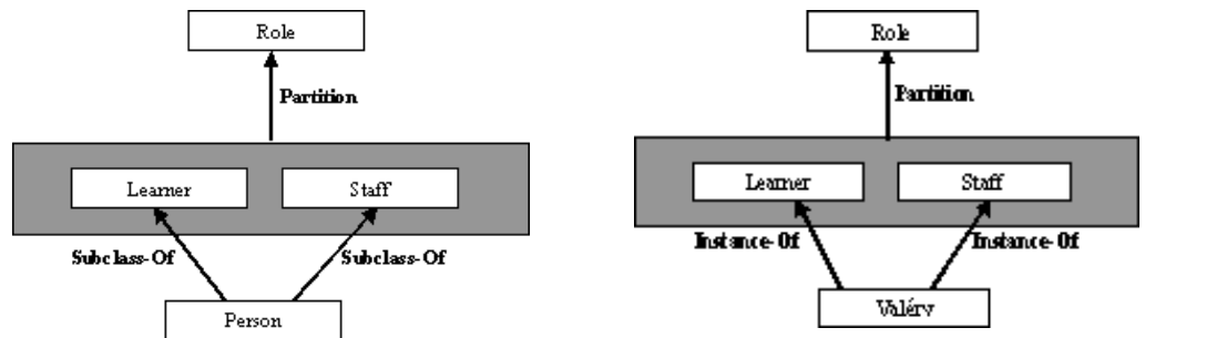
E5 (b) Instances communes à une partition.
