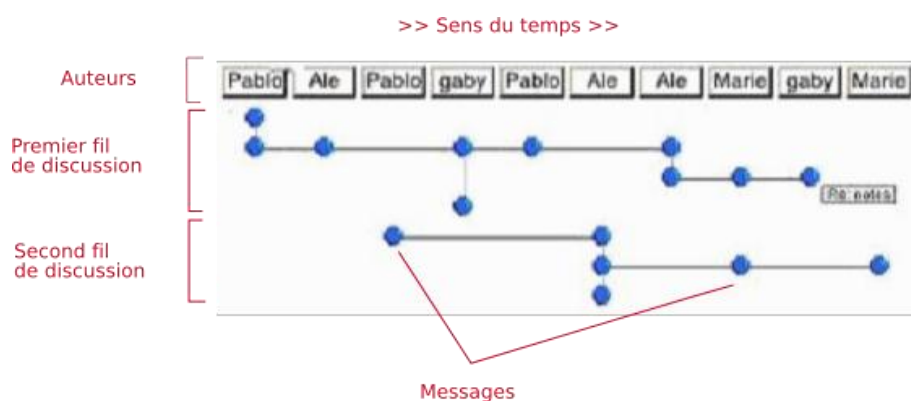
Figure 2. Interface de Reyes (2003) avec les messages apparaissant en fonction de leur fil, du temps et de leur auteur
